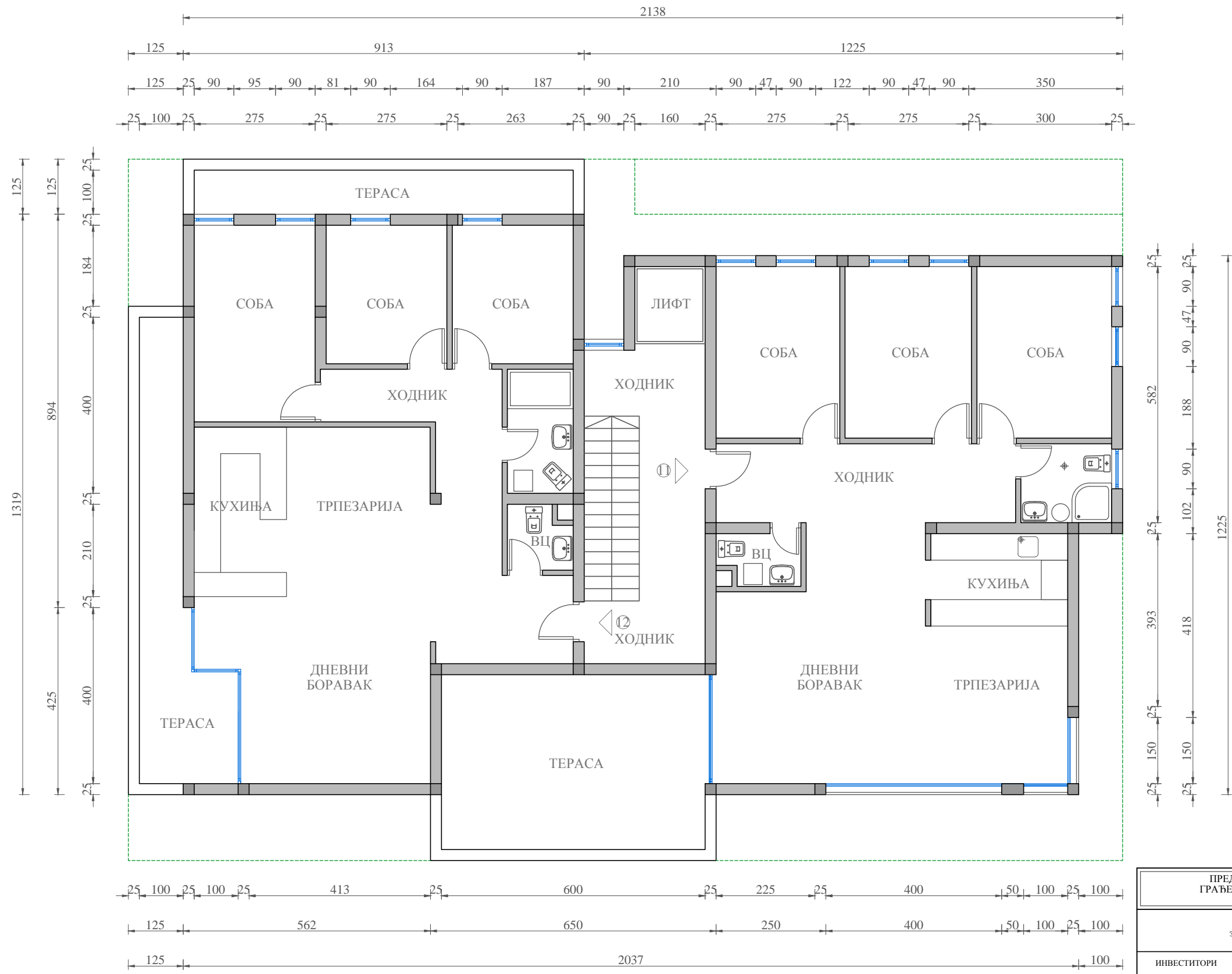
ОСНОВА 4. СПРАТА СТАМБЕНОГ ОБЈЕКТА - P = 1:100
